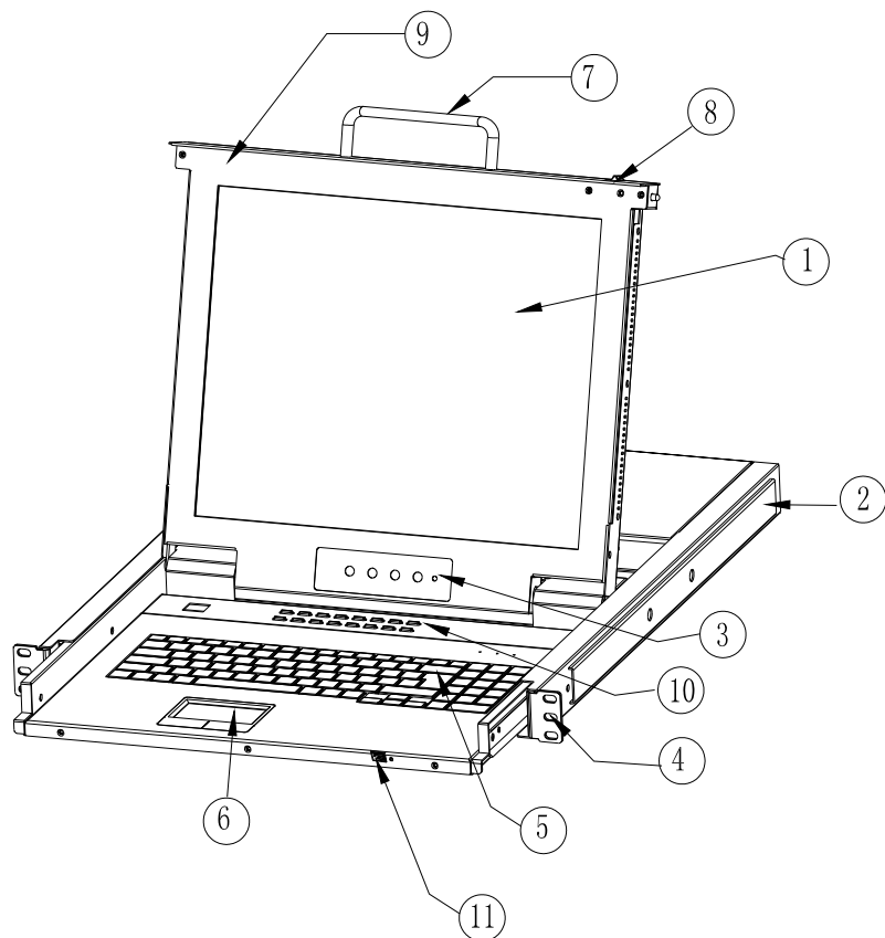
图 1-1.1 前视图
