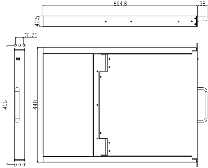
图 1-1.3 19"KVM 尺寸图
