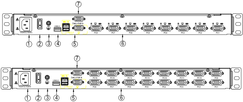
图 1-1.4 后视图
