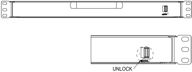
图 2-1.3 解锁方式
